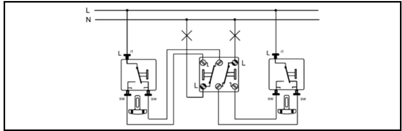
Wiring diagrams
