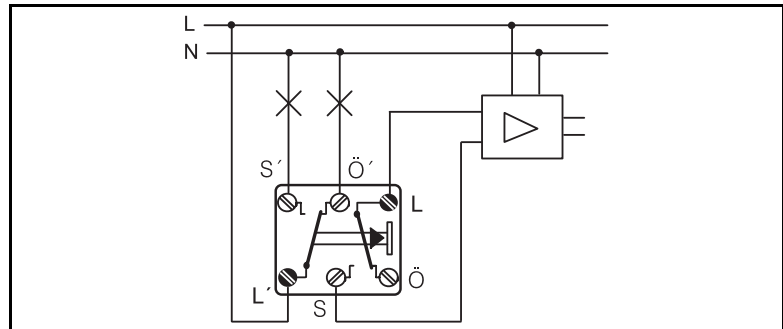
Wiring diagrams 839 W
