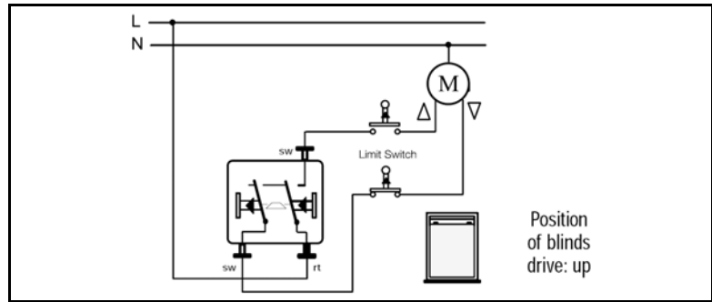
Wiring diagrams 809 VW
