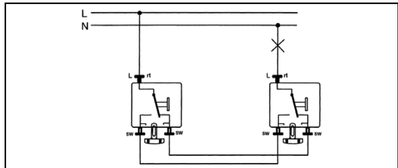
Wiring diagrams
